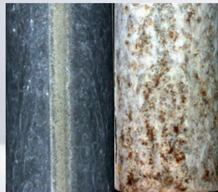
Magnelis® ZM310 Stückverzinkt geschweißt und nachbehandelt zyklischer Korrosionstest (3CT) (VDA 621-415) nach Testzeitraum von 33 Wochen
